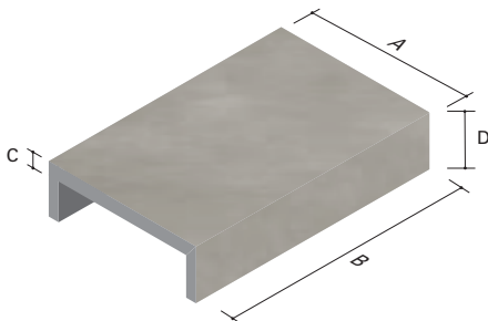
Abdeckplatte
